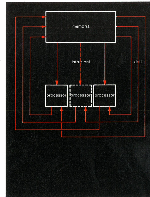
Fig. 8 - Multiprocessor, ovvero flusso multiplo di istruzioni e di dati.
