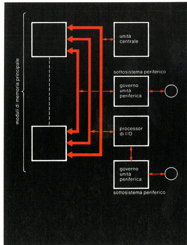
Fig. 2 - Struttura logica con connessione del tipo « canale alla memoria ».
