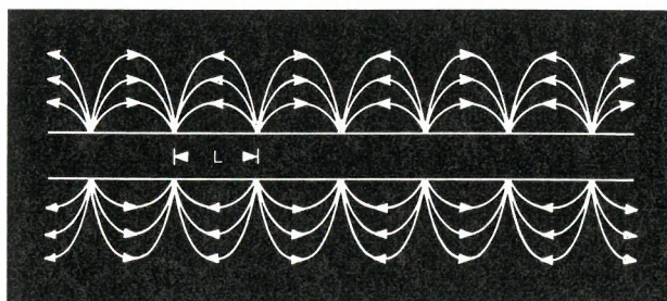
Fig. 5 - Campo magnetico generato da una registrazione del tipo di Fig. 3b).
