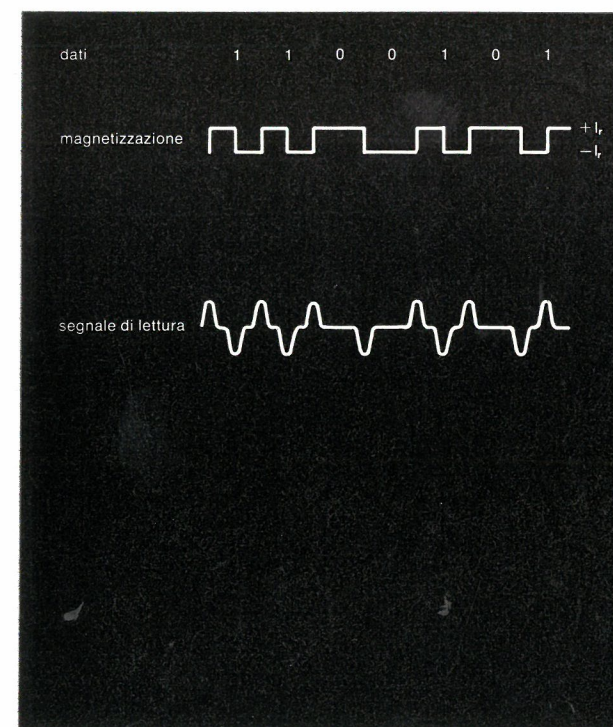
Fig. 12 - Registrazione e lettura col codice PE bifase (o a due periodi).
