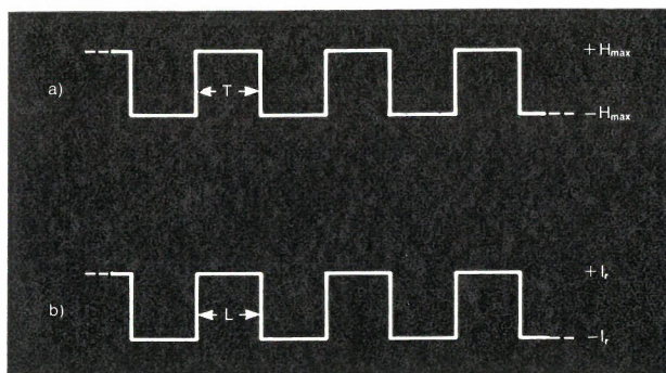
Fig. 3 - Registrazione di un'onda quadra: a) andamento temporale del campo magnetico; b) andamento spaziale della magnetizzazione ( L = vT ).
