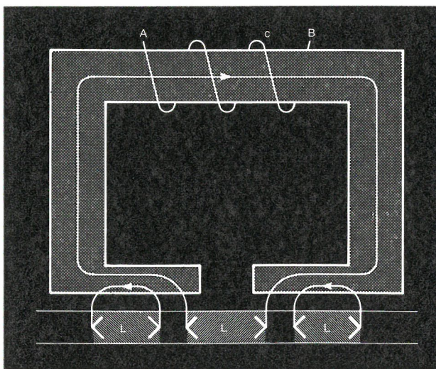
Fig. 6 - Campo magnetico nella testina di lettura.
