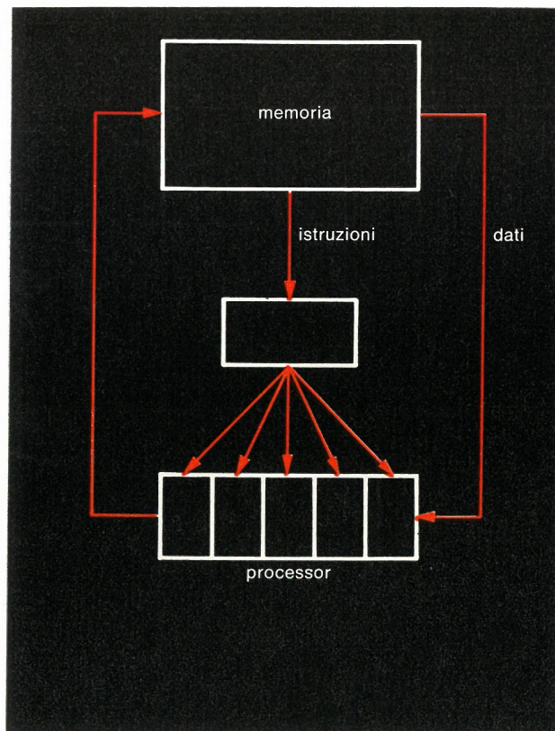
Fig. 5 - Pipeline processor, ovvero flusso multiplo di istruzioni e singolo di dati.
