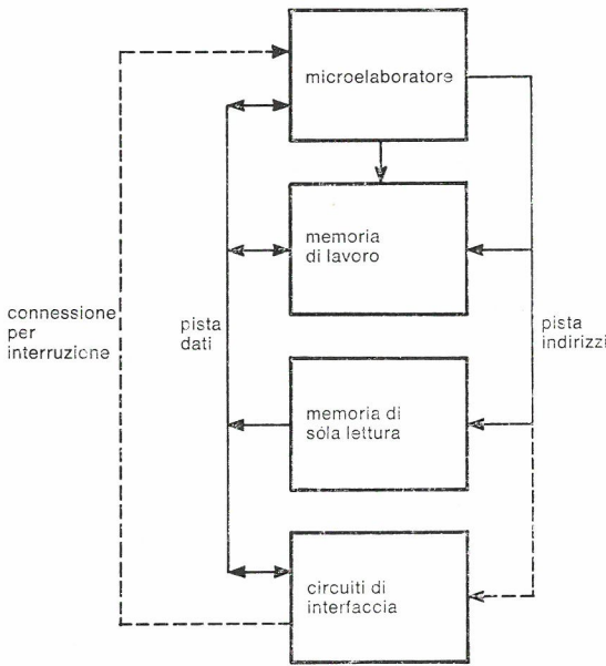
Fig. 1 - Microelaboratore e dispositivi integrati associati.
