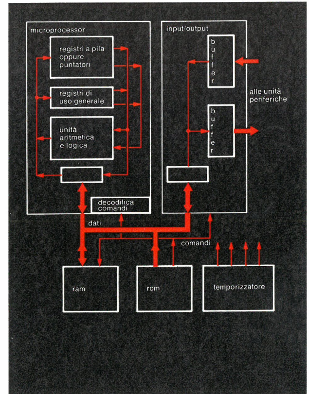
Fig. 9 - Schema logico di un micro sistema di elaborazione composto da 5 «chip».
