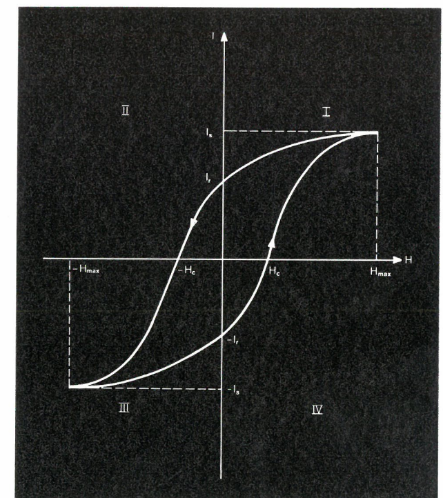
Fig. 2 - Ciclo di isteresi per un materiale ferromagnetico.
