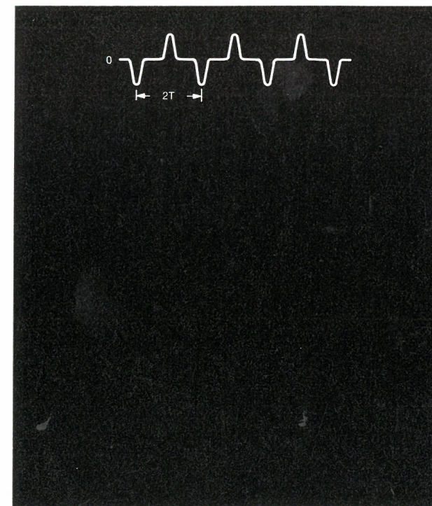
Fig. 7 - Differenza di potenziale in una testina di lettura.
