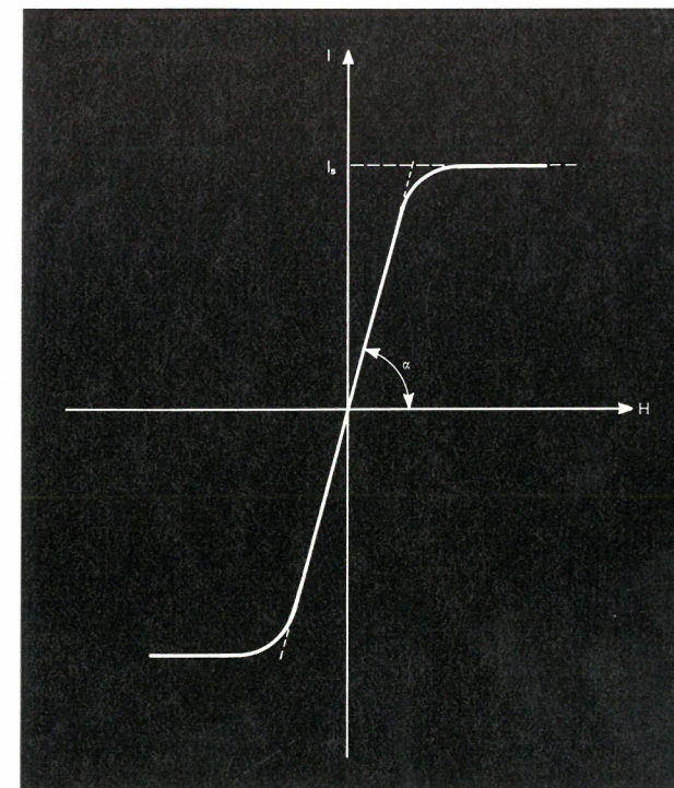
Fig. 9 - Relazione tra I e H in un materiale ferromagnetico dolce ( H_c = 0 ).
