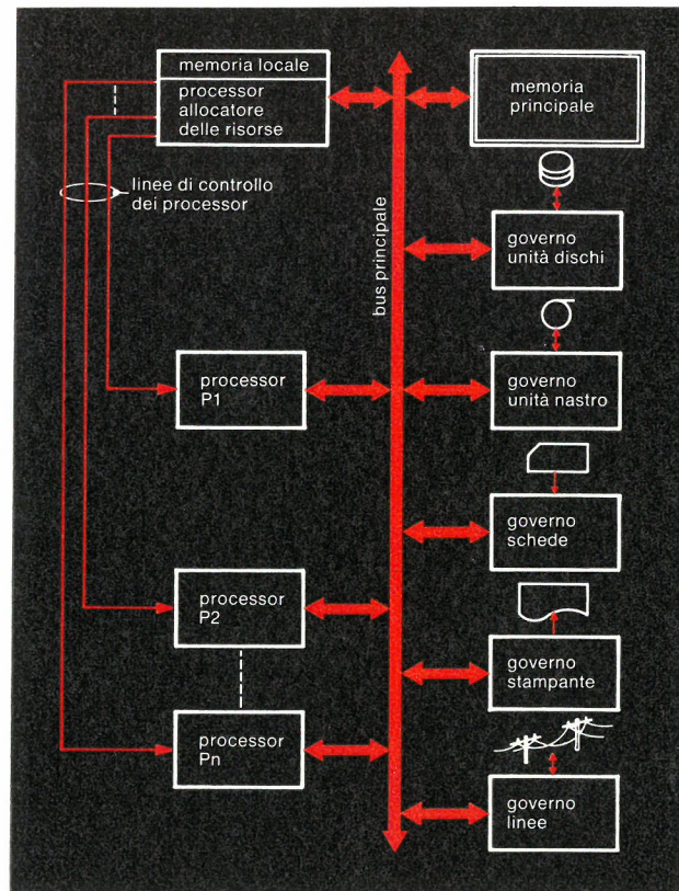
Fig. 10 - Insieme di processor di tipo generalizzato, fra loro connessi mediante un bus, controllati da un processor pilota, comunicanti con la memoria e le unità periferiche.
