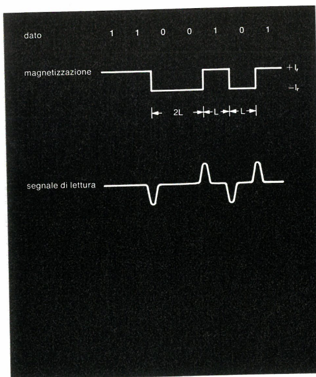
Fig. 10 - Registrazione e lettura NRZ.
