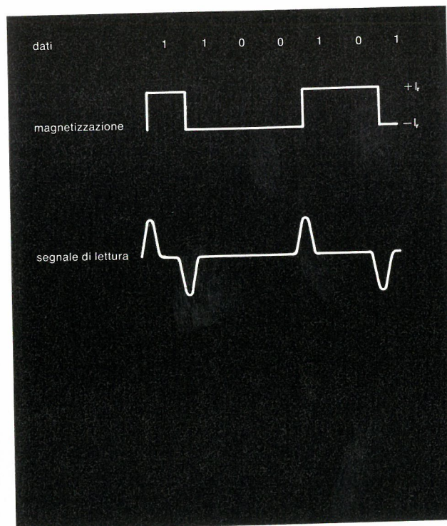
Fig. 11 - Registrazione e lettura NRZI.
