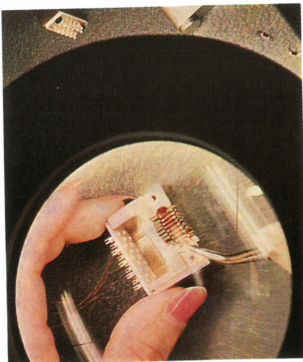
Fig. 14 - Montaggio di una testina di registrazione a nove tracce per nastri magnetici. (Stabilimento di Caluso della Honeywell Information Systems Italia).
