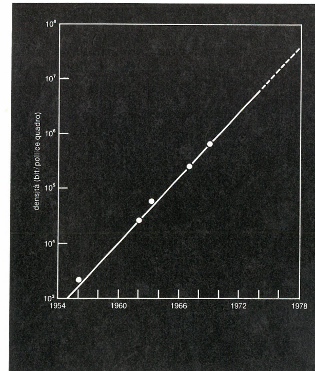
Fig. 16 - La densità superficiale di informazioni nelle memorie elettromeccaniche di massa. I punti corrispondono ai prodotti più significativi annunciati nel corso del tempo.
