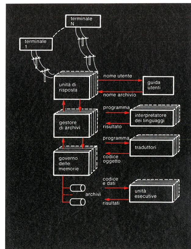
Fig. 11 - Sistema con « intelligenza » distribuita.
