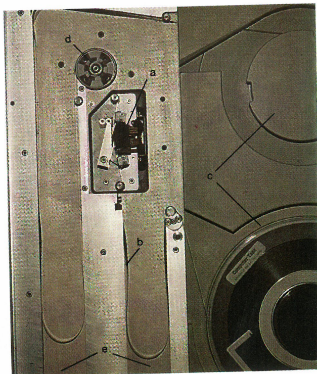
Fig. 15 - Organi di trascinamento e registrazione di una moderna unità a nastro magnetico (progetto e fabbricazione Honeywell Information Systems Italia). a) Testina magnetica, b) Nastro magnetico (lato di registrazione), c) Bobine, d) Rullo di trascinamento del nastro, e) Polmoni pneumatici (per controllare la tensione del nastro).
