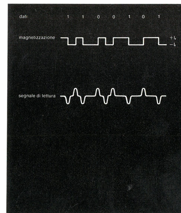
Fig. 13 - Registrazione e lettura col codice PE Manchester.
