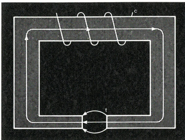
Fig. 4 - Testina di registrazione.
